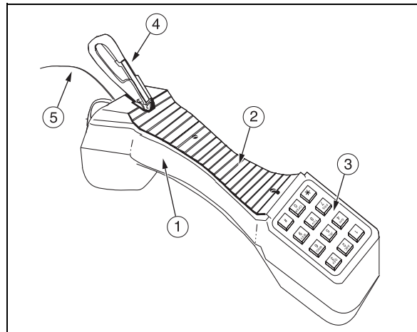
Рисунок 1. Внешний вид
